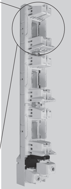
4) Sicherung einsetzen/entnehmen Fuse-link insert/remove
