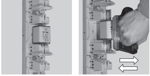
4) Sicherung einsetzen/entnehmen Fuse-link insert/remove
