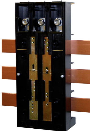
Flexible Positionierungsschiene für Leistungsschalter verschiedener Hersteller Flexible positioning rail for circuit breakers of different manufactures
